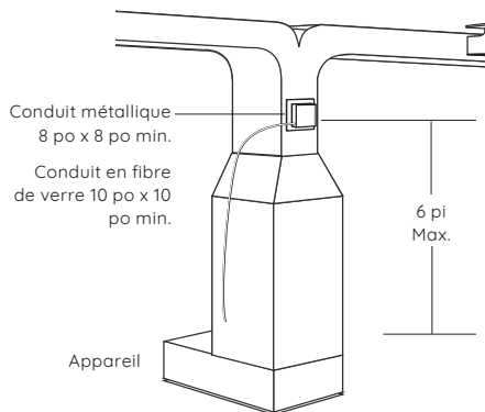
Dégagement pour l'installation
